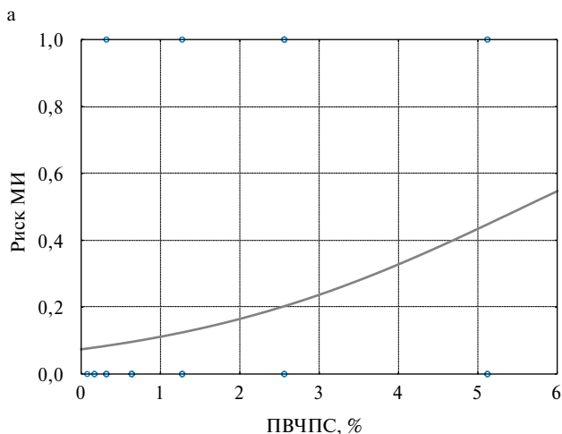
Примечание: Chi-square=7,9, df=1, p=0,005.
